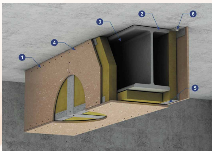
Противопожарная защита металлоконструкций
