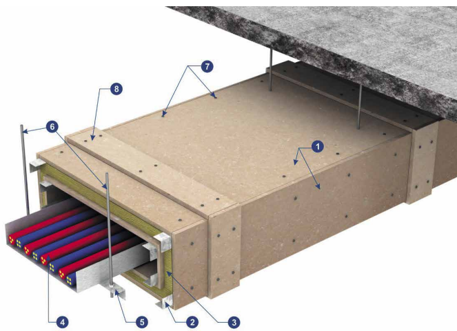
Кабельные каналы
