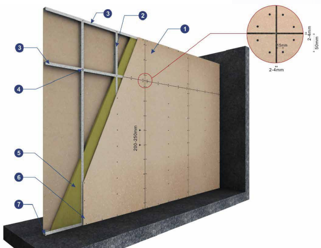
Огнестойкие перегородки
