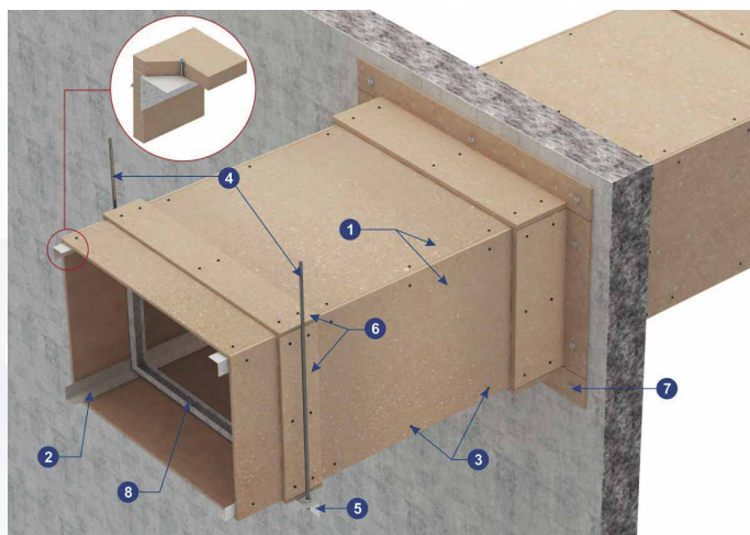
Воздуховоды
