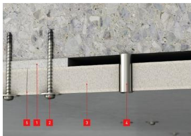
Огнезащита железобетонных конструкций
