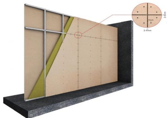
Огнестойкие перегородки, стены и перекрытия
