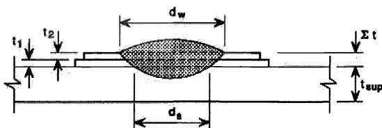
б) присоединение двух листов ( \Sigma t=t_1+t_2 )
