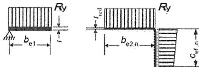
Рисунок Б.6 – Окончательное сечение полки
