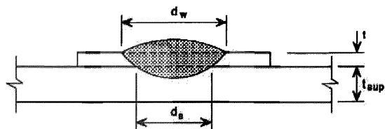
а) присоединение одного листа ( \Sigma t=t )
