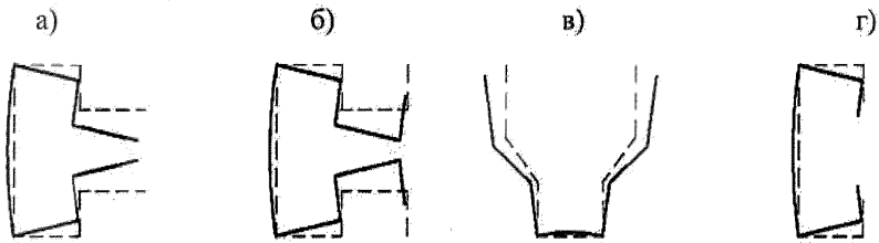
Рисунок 7.6 – Примеры потери устойчивости формы сечения
