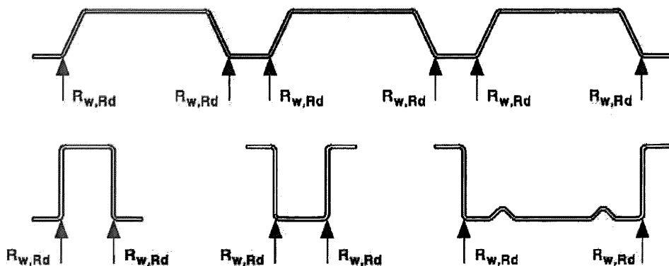
Рисунок 7.22 – Примеры профилей с двумя и более стенками
