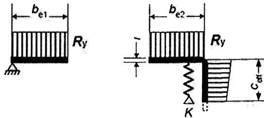
Рисунок Б.2 – Схема к этапу I
