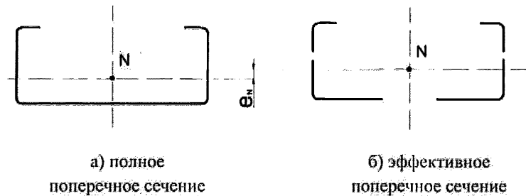
Рисунок 7.15 – Эффективное поперечное сечение при сжатии
