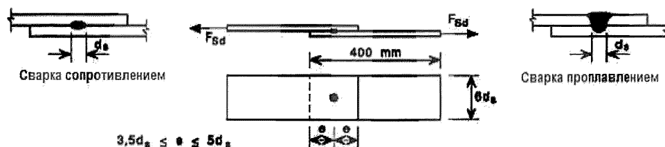
Рисунок 10.2 – Образцы для испытаний на срез сварных точек
