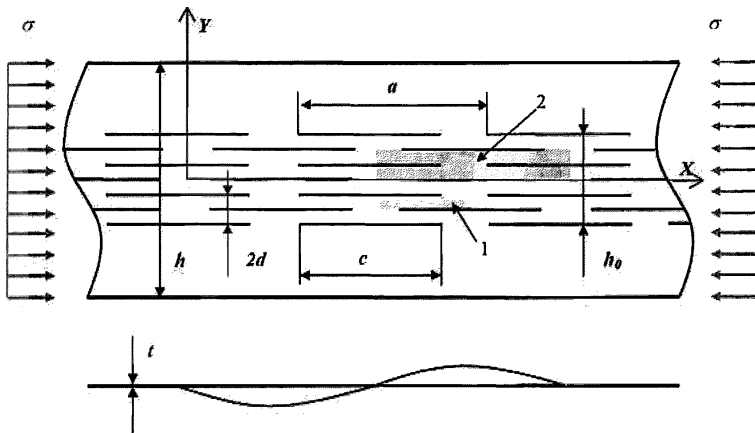
Рисунок 7.24 – Параметры щелевой перфорации термопрофилей
