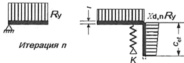
Рисунок Б.5 – Схема к этапу III
