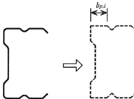
б) идеализированное поперечное сечение
