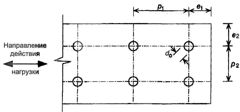
Рисунок 10.1 – Расположение метизов в соединениях
