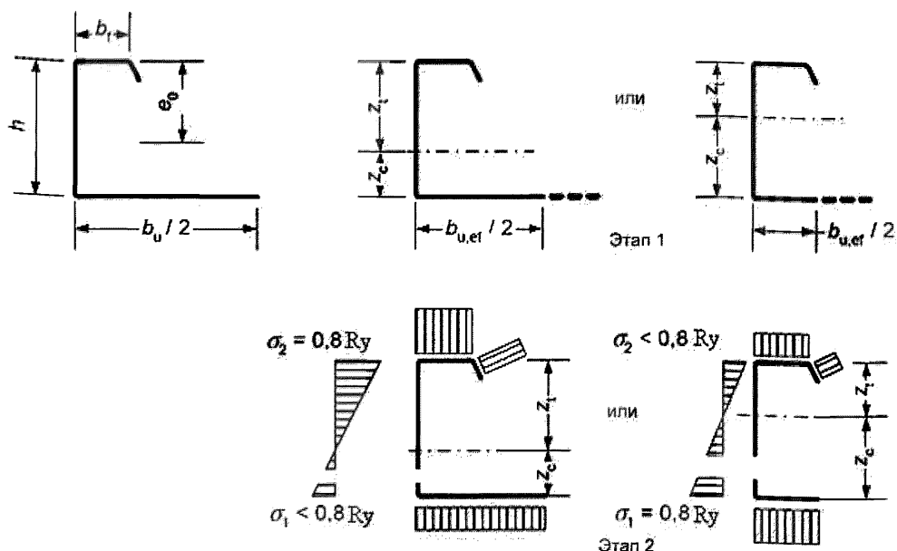
Рисунок 8.2 – Определение предельного момента при сжатой широкой полке
