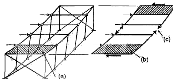
Рисунок А.2 – Работа диафрагмы в здании с плоским покрытием
