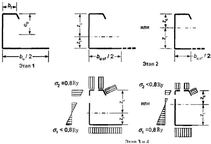
Рисунок 8.3 – Определение предельного момента при растянутой широкой полке
