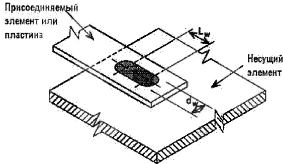
Рисунок 10.5 – Овальная сварная точка
