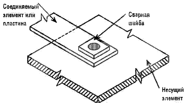
Рисунок 10.3 – Дуговая точечная сварка со сварной шайбой
