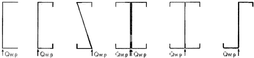
Рисунок 7.21 – Примеры сечений профилей с одной стенкой
