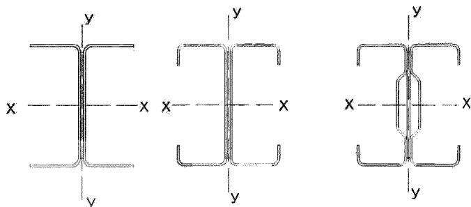
Рисунок 7.19 – Сечения сплошных стержней колонн и стоек
