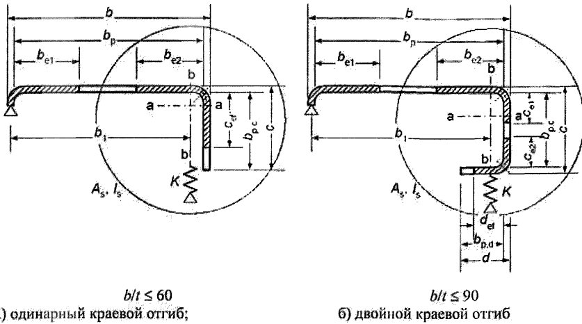
Рисунок 7.8 – Краевые отгибы
