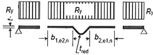
Рисунок Б.12 – Окончательное расчетное сечение полки
