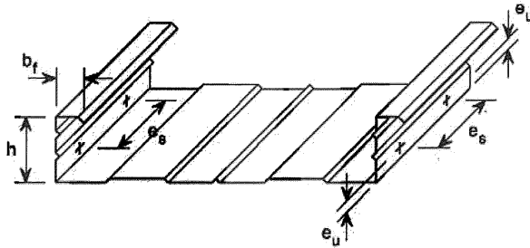
Рисунок А.5 – Расположение метизов в продольном стыке
