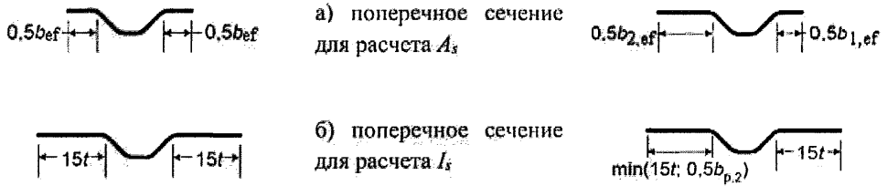
Рисунок 7.10 – Включение в ребро жесткости примыкающих участков полки
