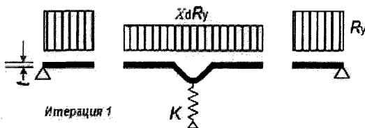
Рисунок Б.10 – Схема к этапу III
