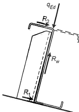
Рисунок А.1 – Реакции на опоре
