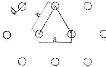
Рисунок 7.23 – Схема расположения отверстий в перфорированном настиле
