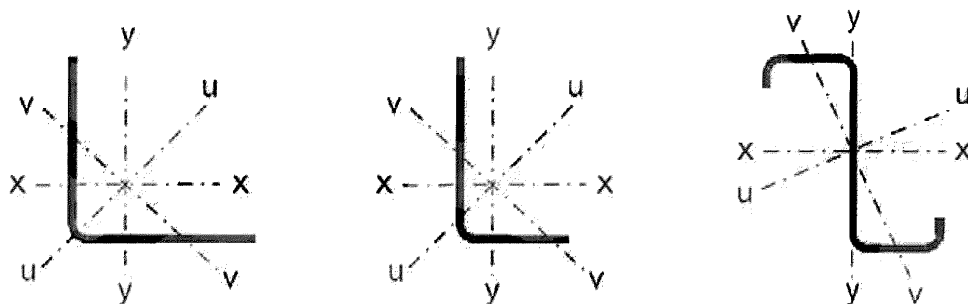
Рисунок 7.2 – Обозначения осей
