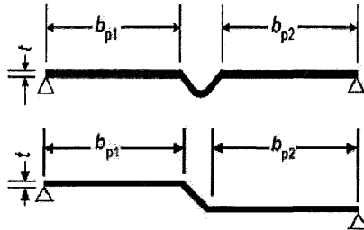
Рисунок Б.7 – Схема полного сечения полки (стенки)
